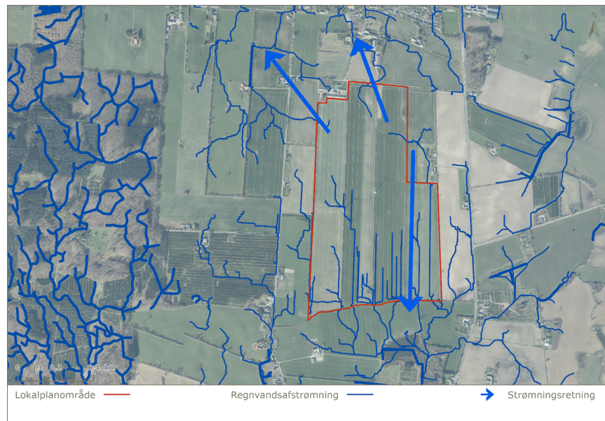
Figur 14. Eksisterende regnvandsafstrømning
