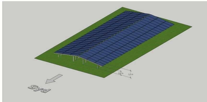
Figur 6. Illustration af fixed-tilt E/W.
