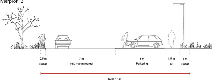
Tværprofil 2
